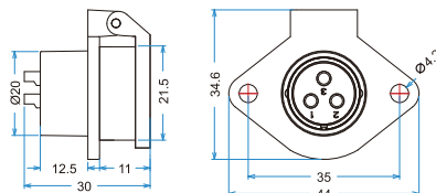
插座 SX (外型尺寸图) SX socket ( dimensions figure )
