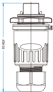
产品外形尺寸图 dimensions figure
