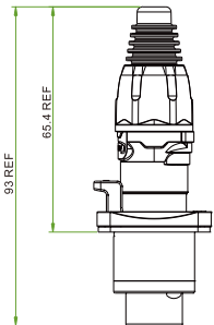
产品外型尺寸图 dimensions figure
