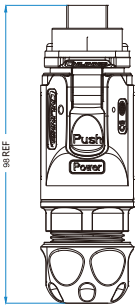
产品外型尺寸图 dimensions figure
